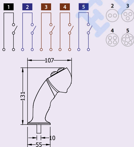
■ EET Esquema eléctrico / Electrical diagram
