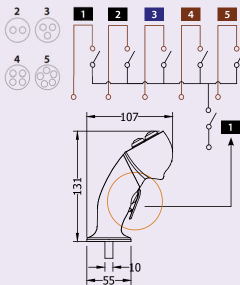
■ EEIT Esquema eléctrico / Electrical diagram
